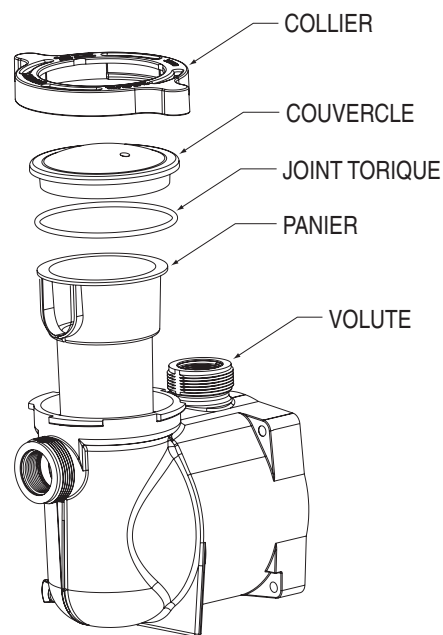
Ensemble du boîtier de la crépine
